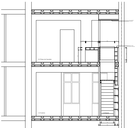
Querschnitt
